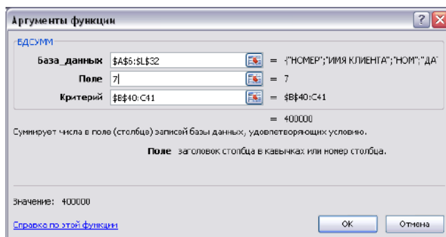
Рис. 10.10. Диалоговое окно аргументов функции БДСУММ
