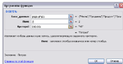
Рис. 11. 35. Диалоговое окно функции БИЗВЛЕЧЬ для задания 16
