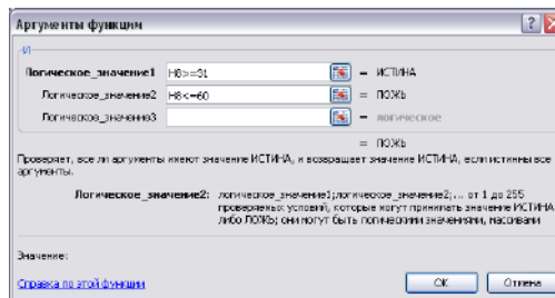
Рис. 10. 4. Диалоговое окно аргументов функции И
