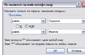
Рис. 11. 7. Пользовательский автофильтр
