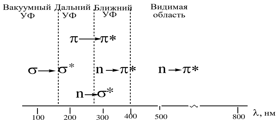
Рис. 7.11. Спектральные области и соответствующие им типы электронных переходов
