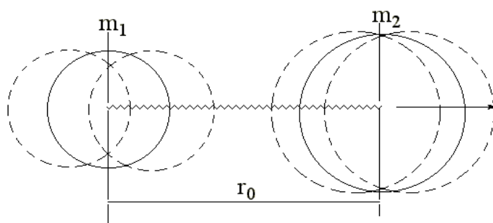
Рис.7.6. Модель колебания двухатомной молекулы.
