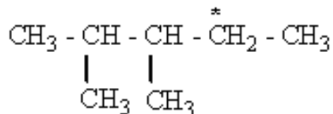
2,3-диметилпентан
